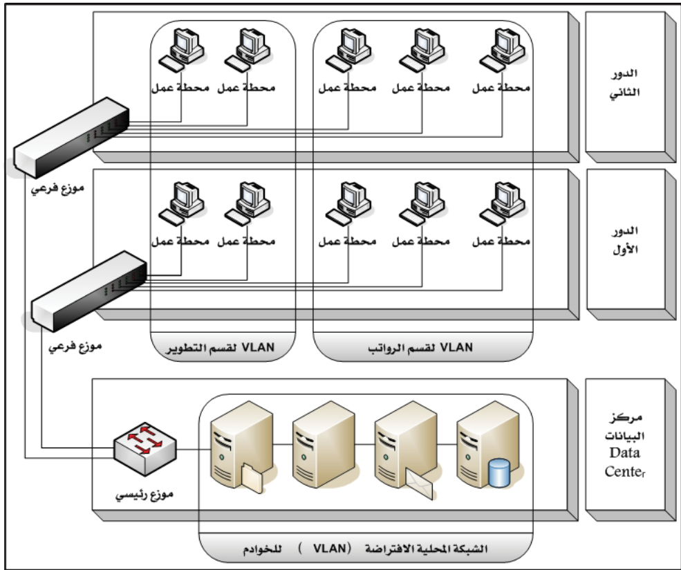
الشكل (٧-٤): الشبكات المحلية الافتراضية (VLANs)
