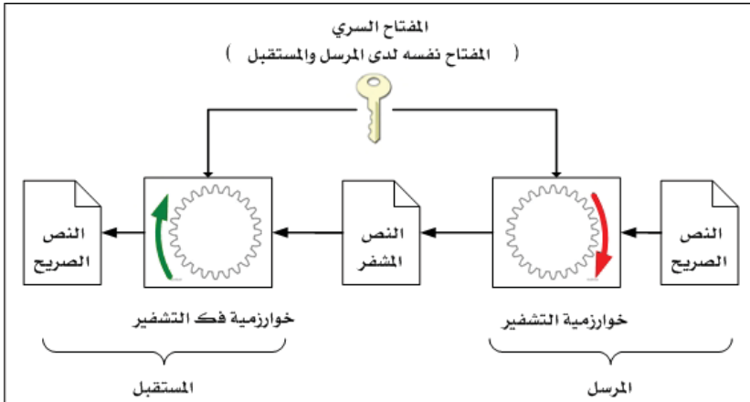
الشكل (٤-٢): التّشفير المتناظر
