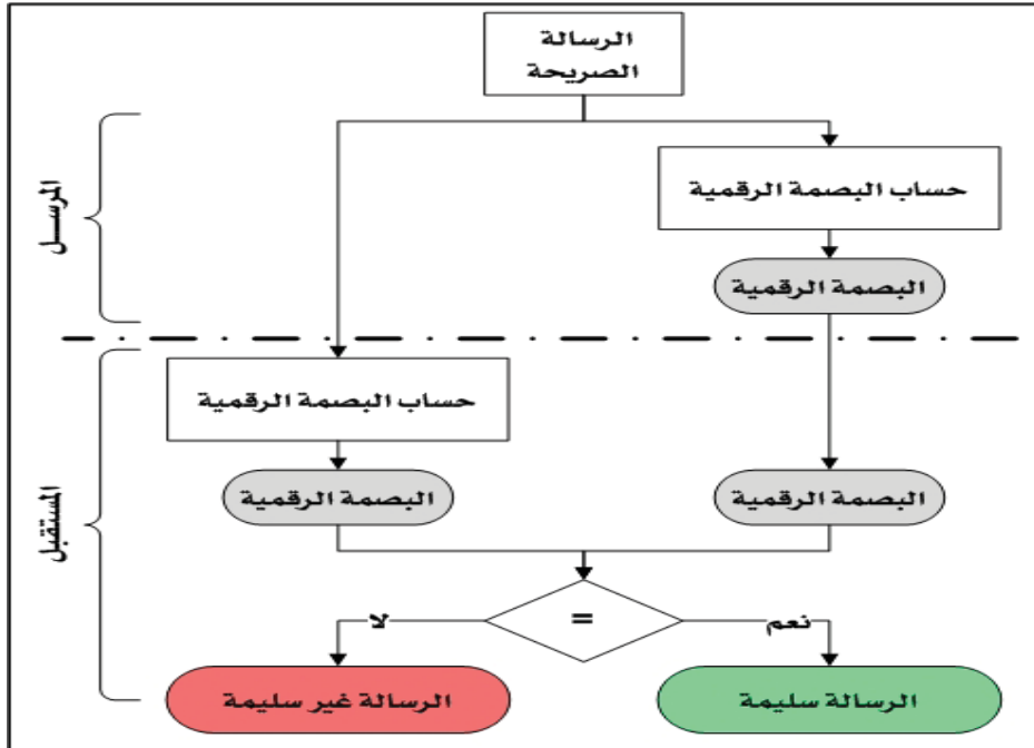
الشكل (٤-١٩): التحقق من سلامة وتكامل الرسالة باستخدام البصمة الرقمية
